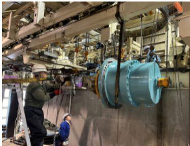
【整備画像】ゴンドラリフト 減速機OH
